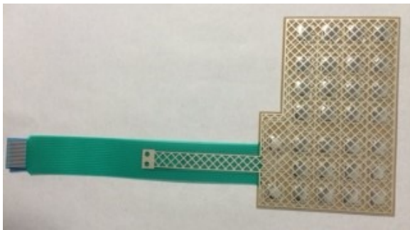
P/N 001-00117: Keypad
